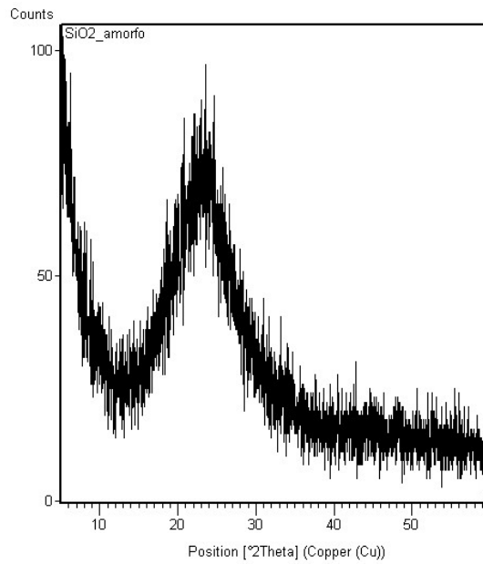
Figura 11. Difractograma del vidrio ( \text{SiO}_2 )
