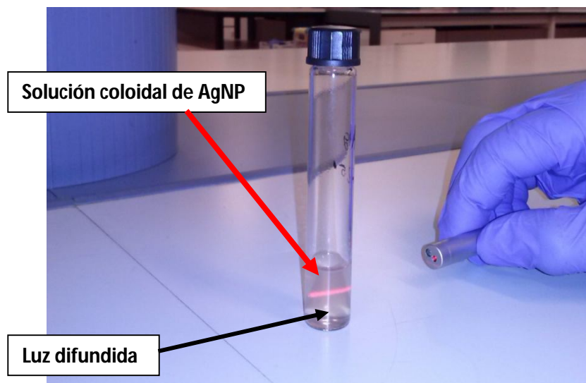
Figura 2. Difusión de la luz del puntero laser por las AgNP
